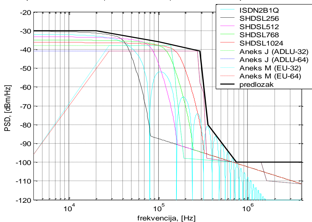
Slika 5.6.4 Frekventijski predložak za odlazni smjer prijenosa (duge pretplatničke linije) za ADSL preko ISDN (aneks B).
